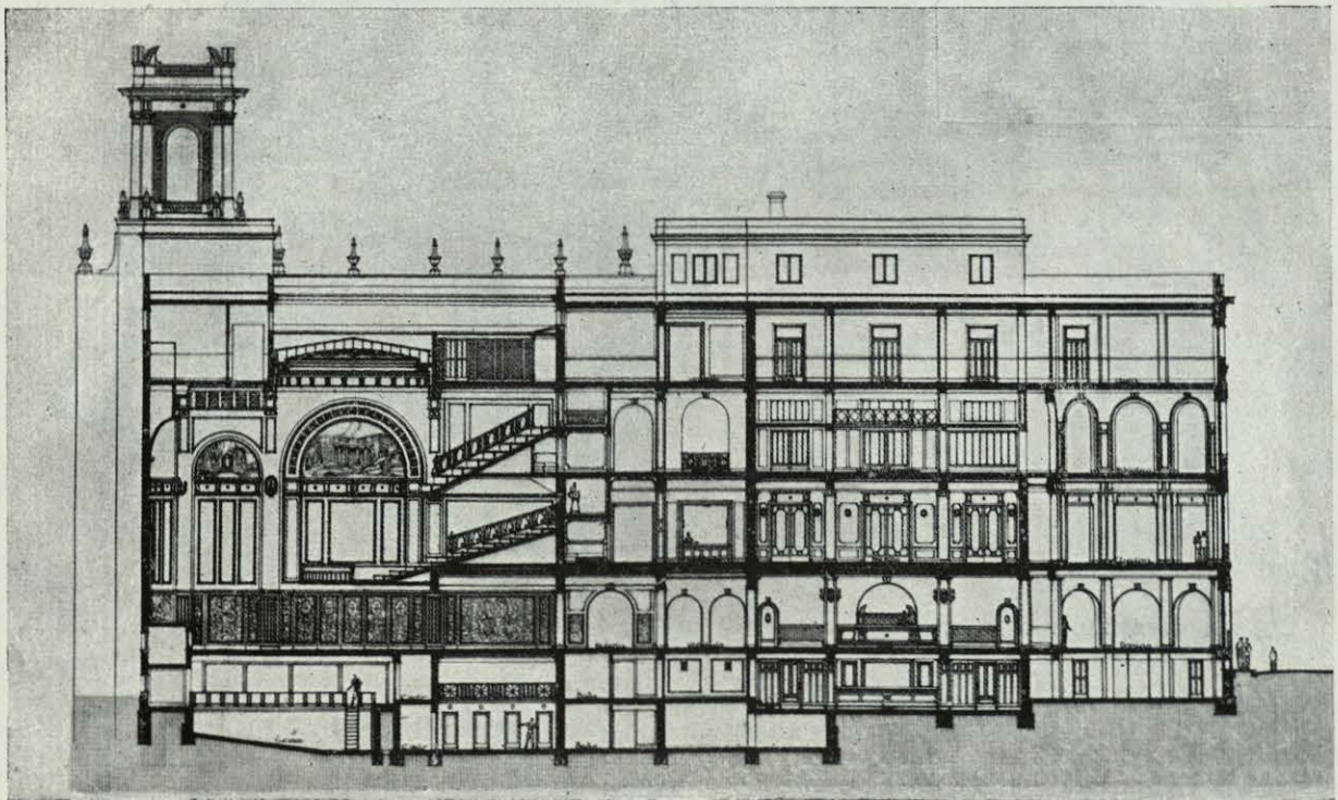
FACHADA Y SECCIÓN LONGITUDINAL.
